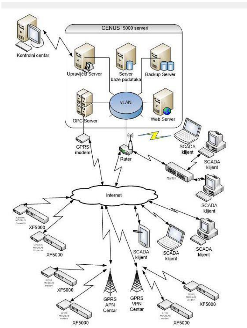
Слика 1. Општа шема комуникације у систему CENUS 5000
