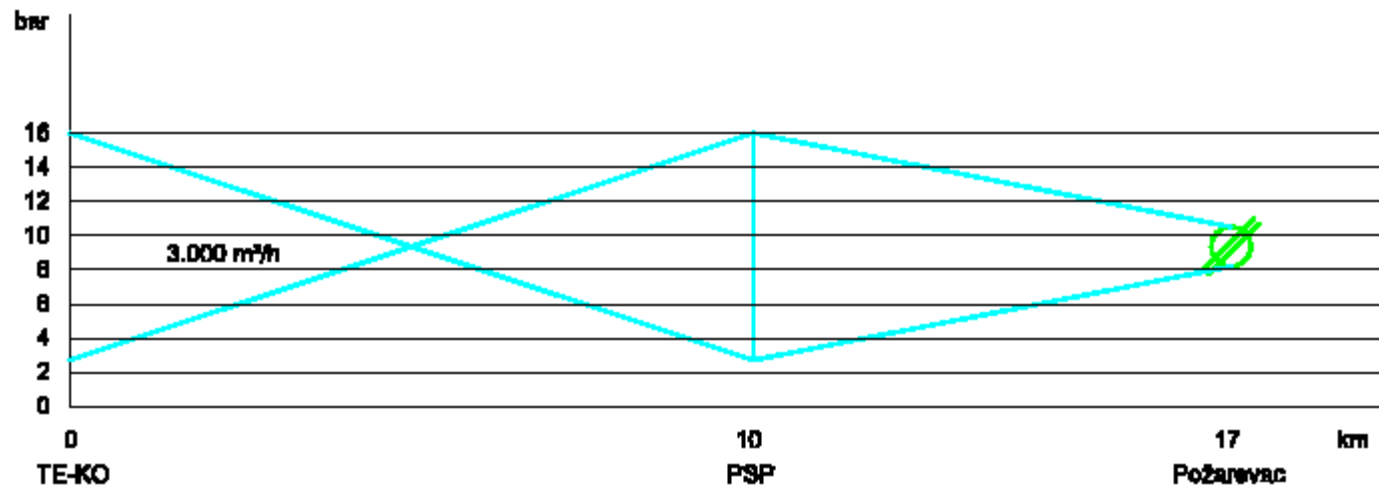
PIEZOMETARSKI DIAGRAM - 3
