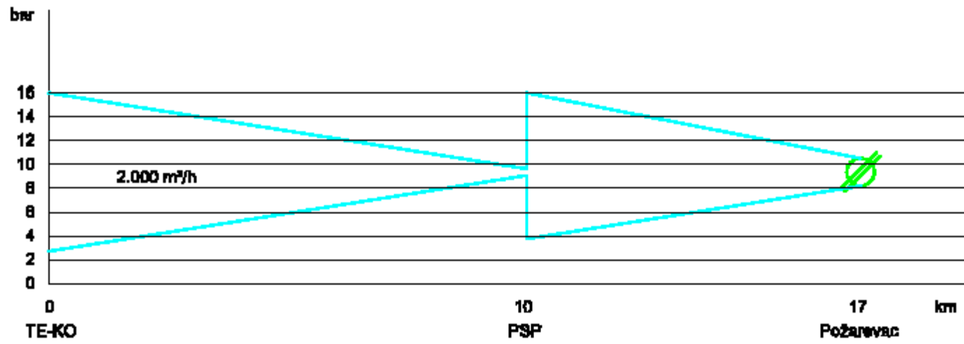
PIEZOMETARSKI DIJAGRAM - 2
