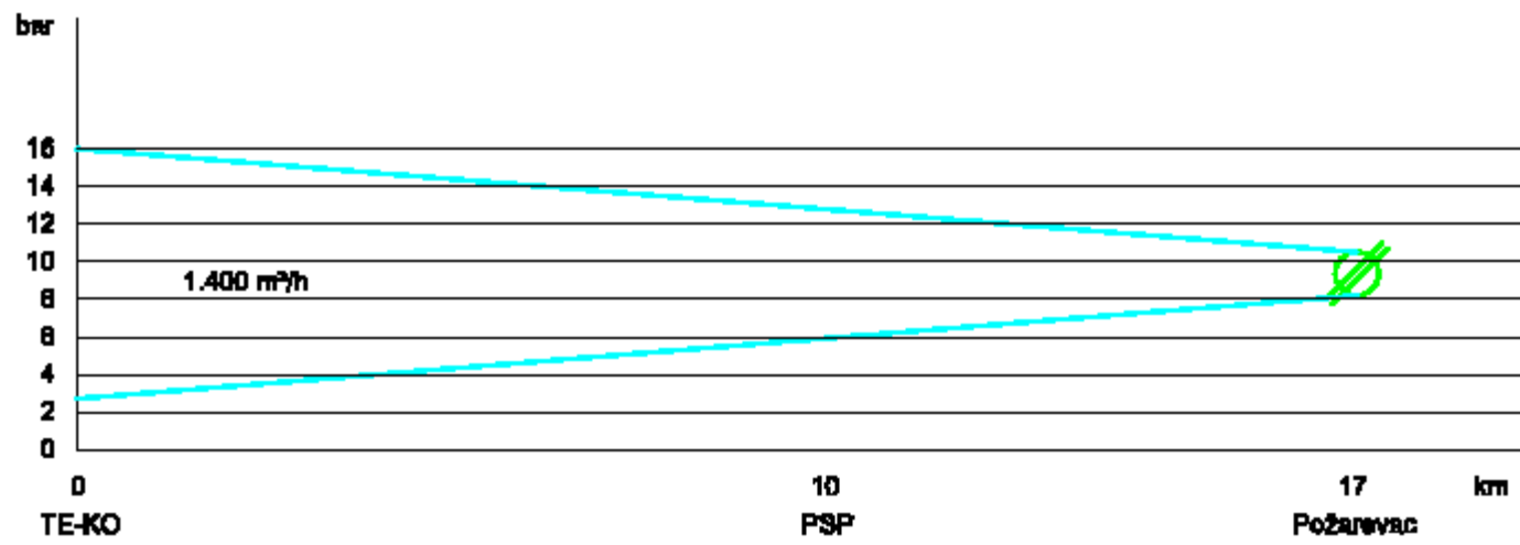
PIEZOMETARSKI DIJAGRAM - 1
